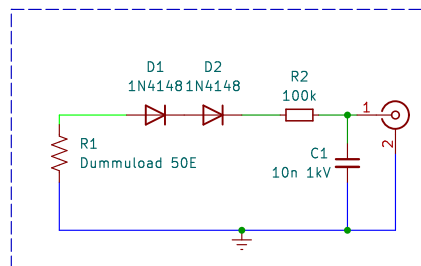
Dummyload med udtag
